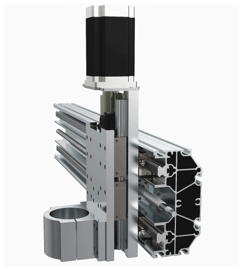
CNC-X-Axis Alu Profile 200×96
